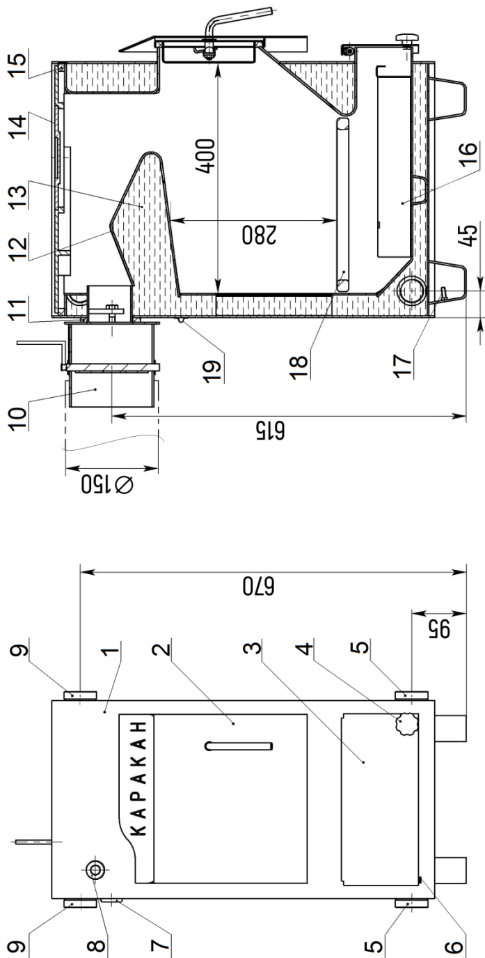
Рисунок 1. Устройство котла. Базовая комплектация
