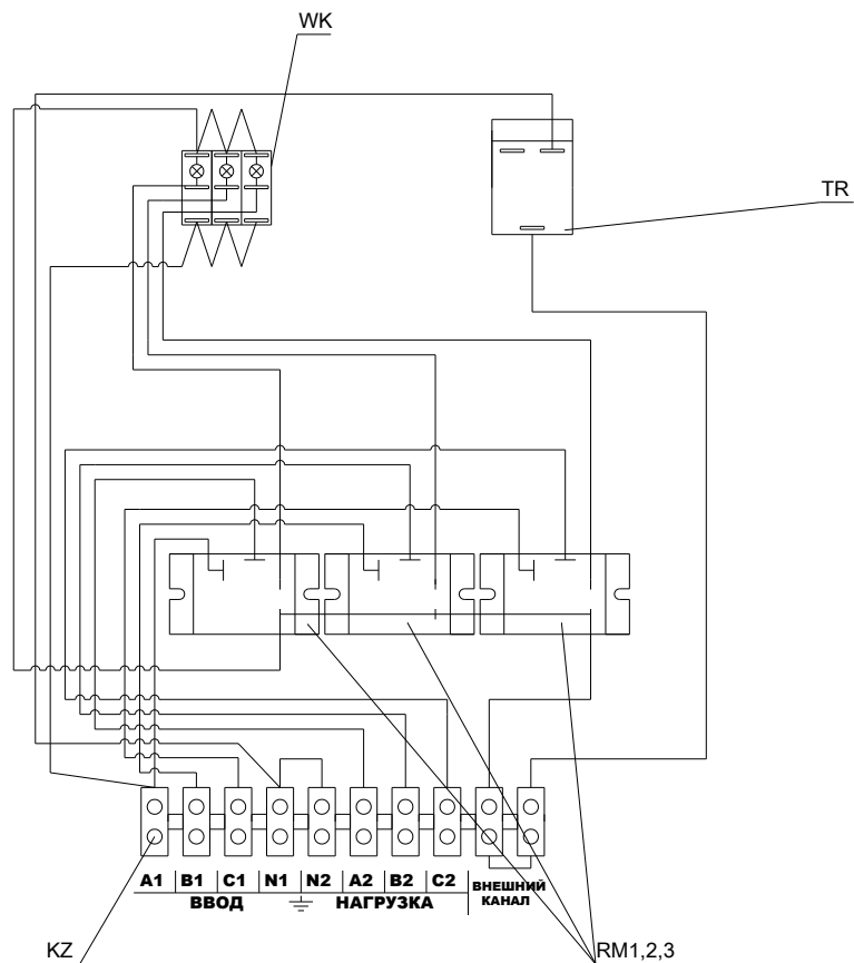
Рис.2 Схема монтажная.
