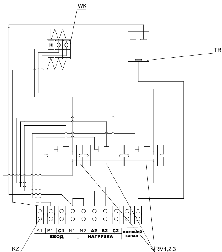
Рис.2 Схема монтажная.
