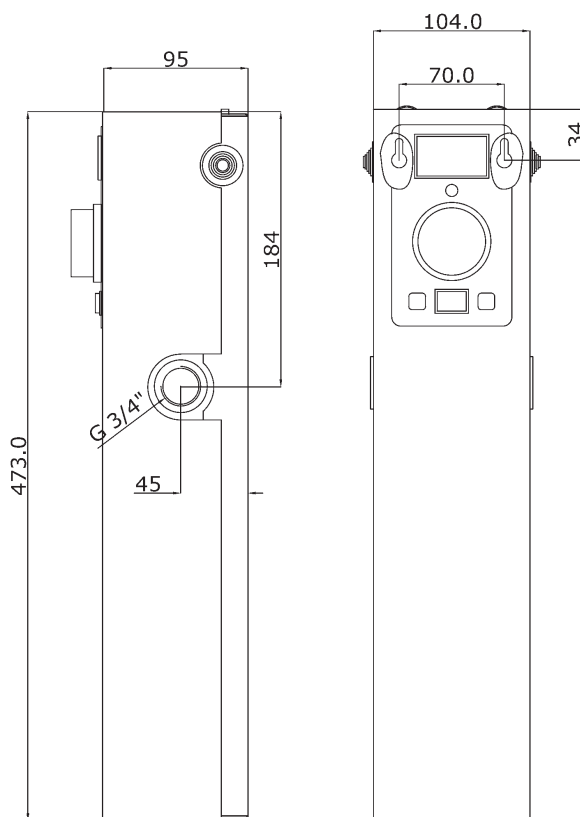
Рис. 7. Монтажные размеры.
