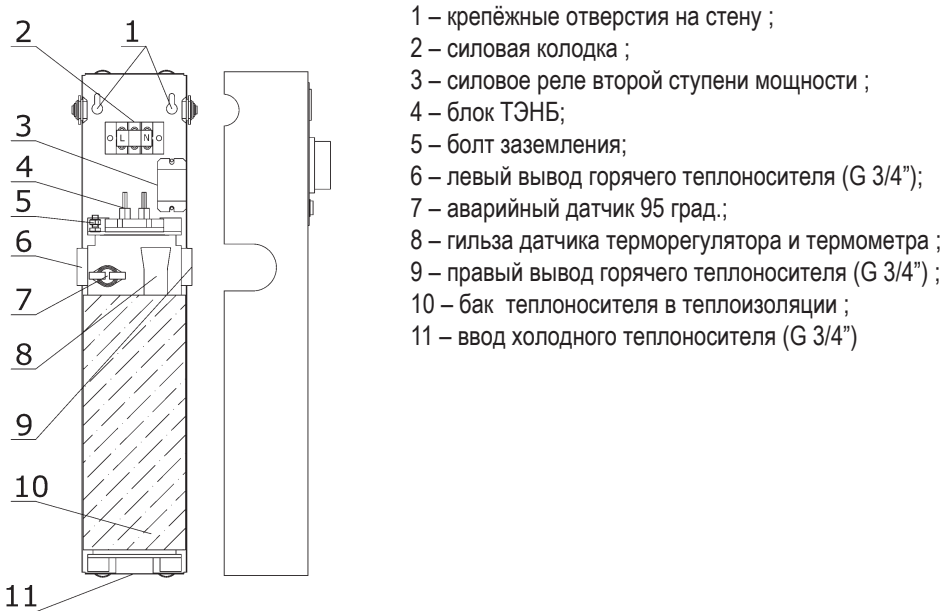
Рис. 3. Устройство электрокотла (крышка снята)
