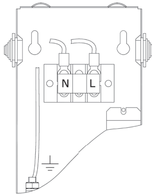
Рис. 6. Подключение электрокотла к сети.
