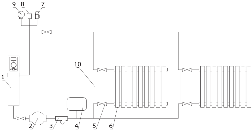
Рис. 5. Упрощенная схема подключения электрокотла в отопительную систему с циркуляционным насосом.
