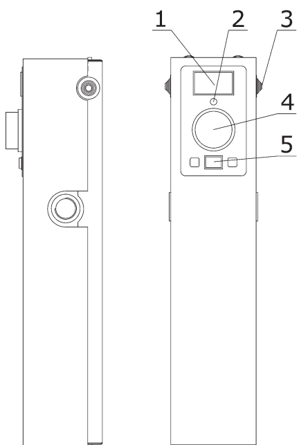
Рис. 2. Устройство электрокотла
