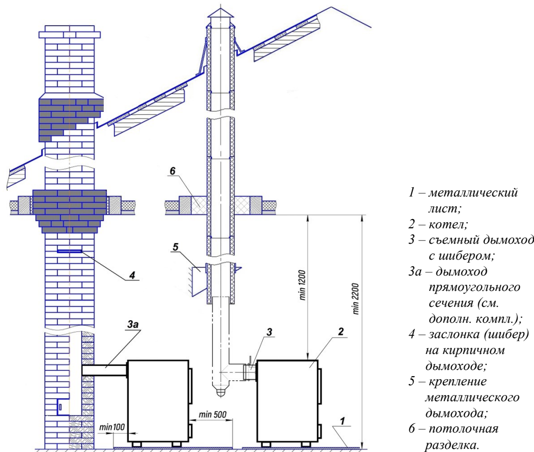
Рисунок 3. Схема установки дымовой трубы
