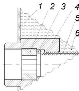
Рисунок 2. Резьбовой фитинг проточного водонагревателя.
